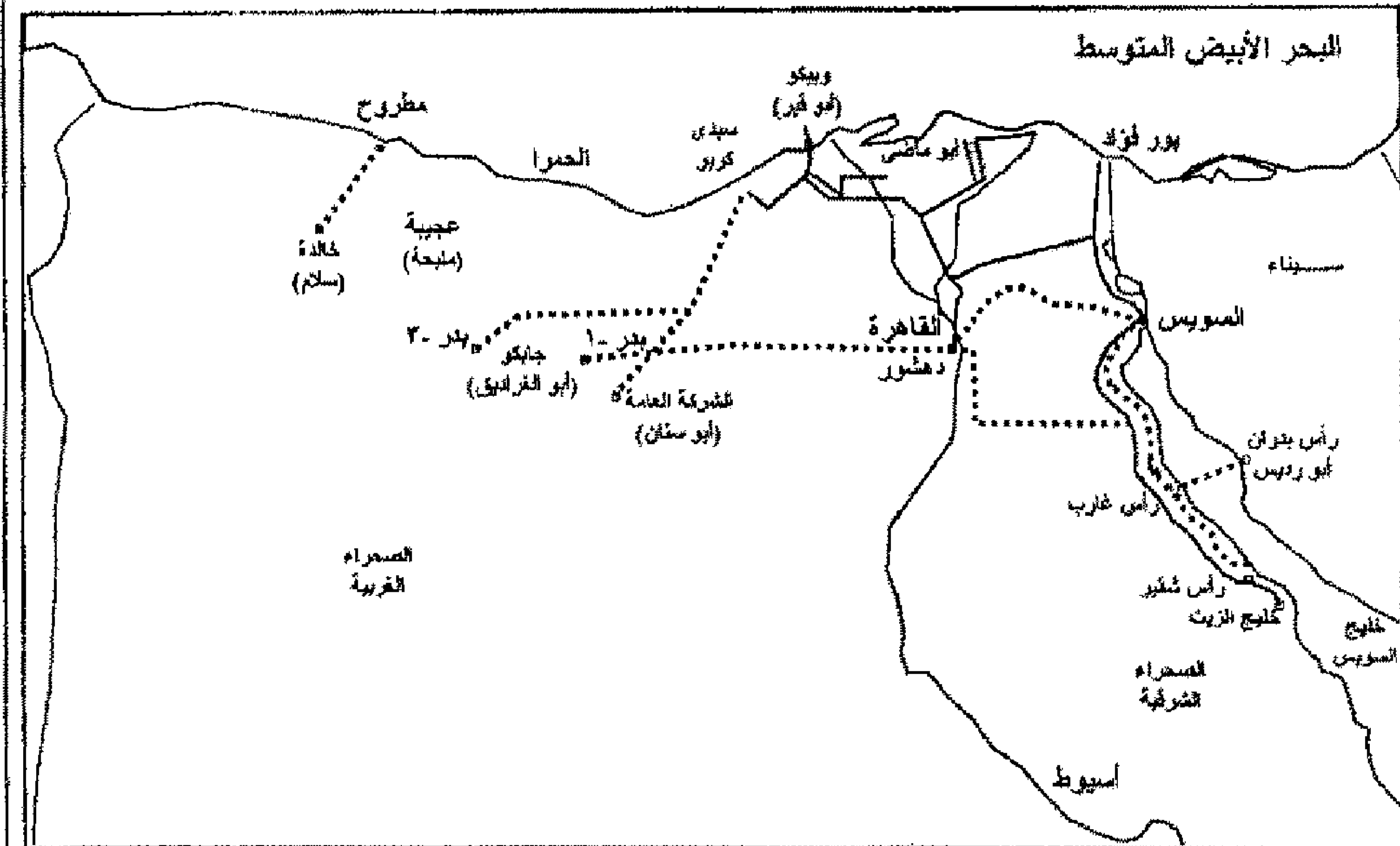
تسهيلات الغاز شبكة أنابيب المنتجين أنابيب الغاز القومية
